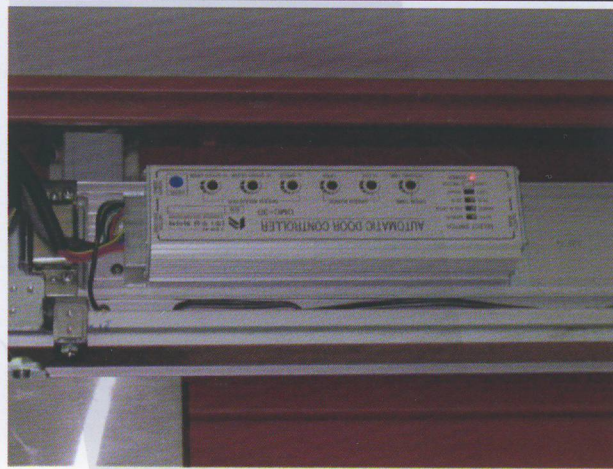
[사진 2] 제어부
