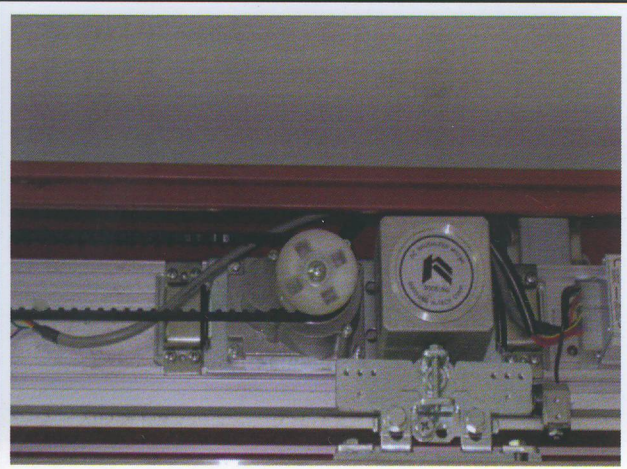
[사진 3] 구동부
